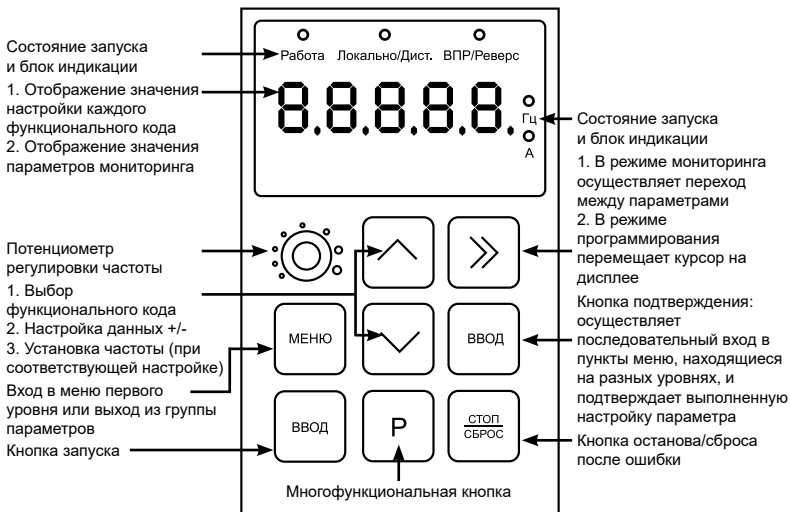
Рисунок 4 – Описание панели управления SDI-KP
