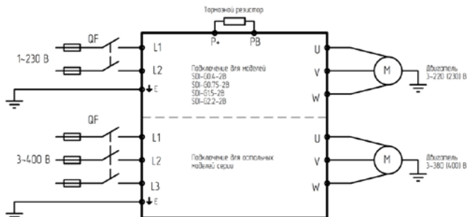
Рисунок 2 – Подключение силовых клемм
