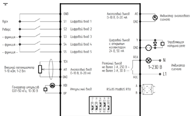
Рисунок 3 – Подключение управляющих клемм
