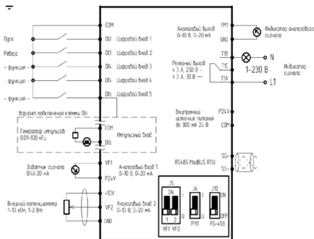
Рисунок 3 – Подключение управляющих клемм
